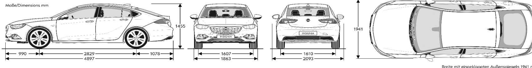
Breite mit eingeklappten Außenspiegeln 1941 mm
