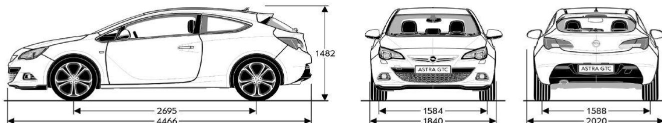
alle afmetingen in mm
